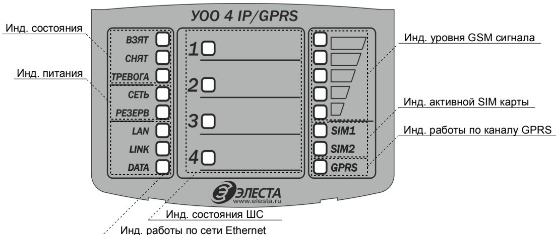
Рис 3. Расположение индикаторов УОО “Юпитер 4 IP/GPRS”
